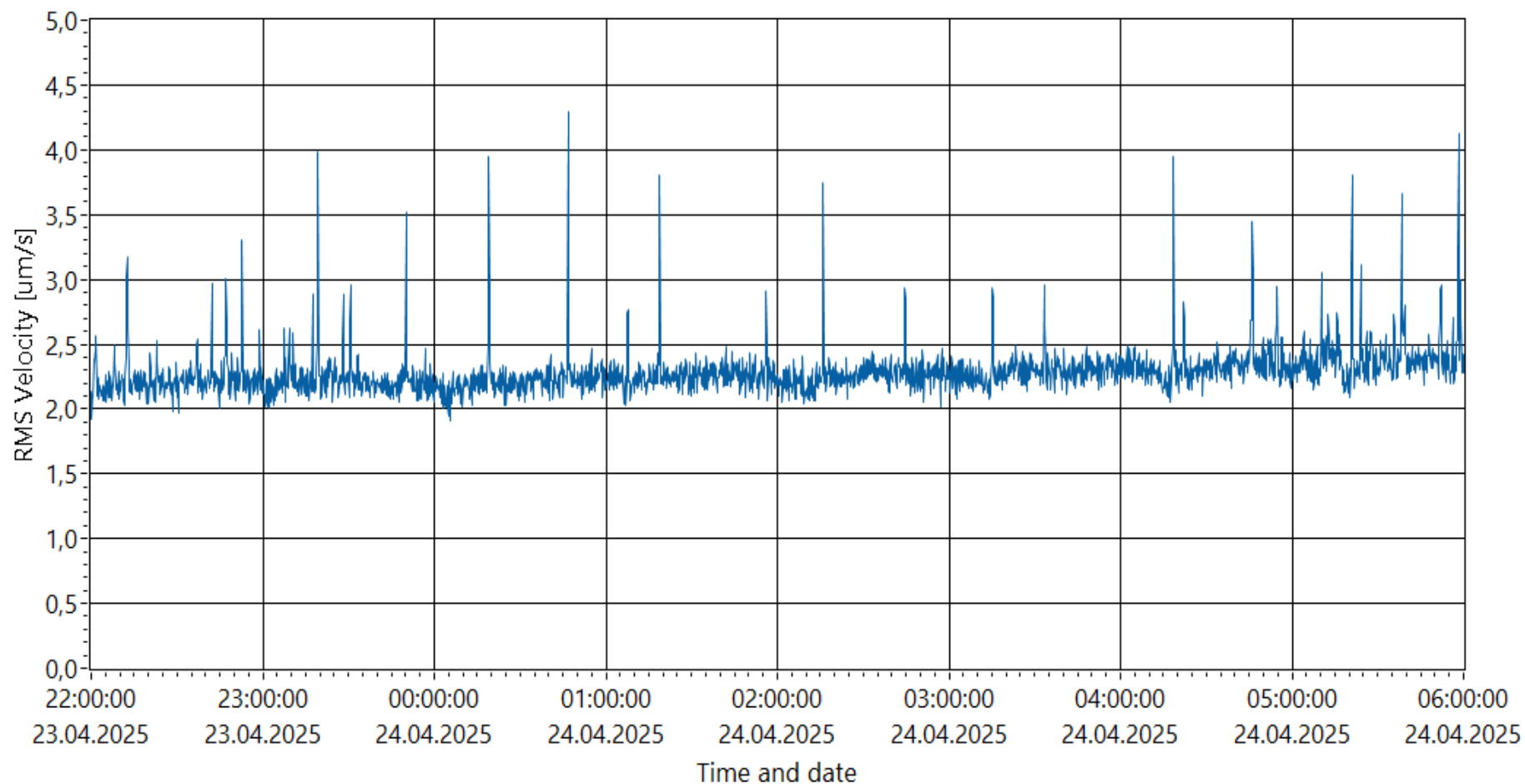
Velocity RMS Values
