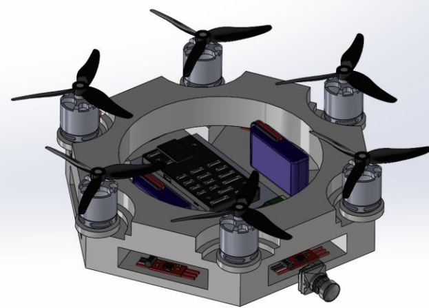
Topologická optimalizace rámu dronu
