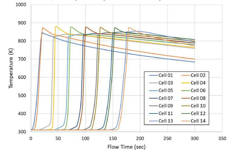
Průběh teploty na jednotlivých člancích
