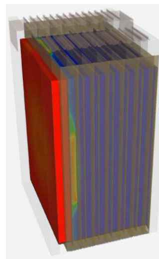
Průběh nail-testu v čase
