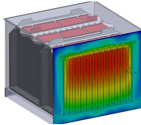
Průběh nail-testu v čase
