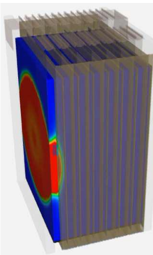
Průběh nail-testu v čase
