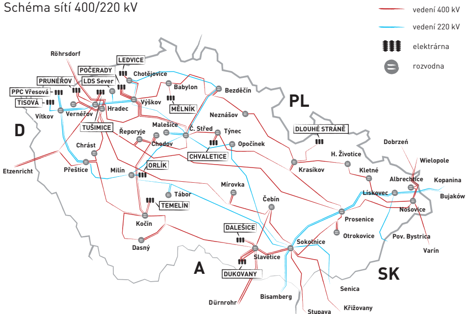
Schéma sítí 400/220 kV
