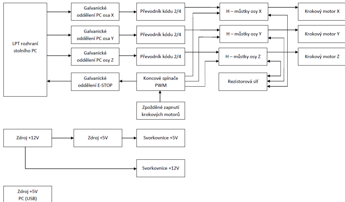
Obrázek 1: Blokové schéma
