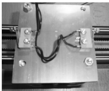
Obrázek 3: Koncové spínače
